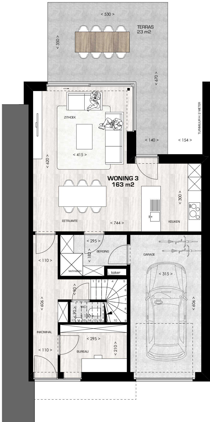
GELIJKVLOERS
