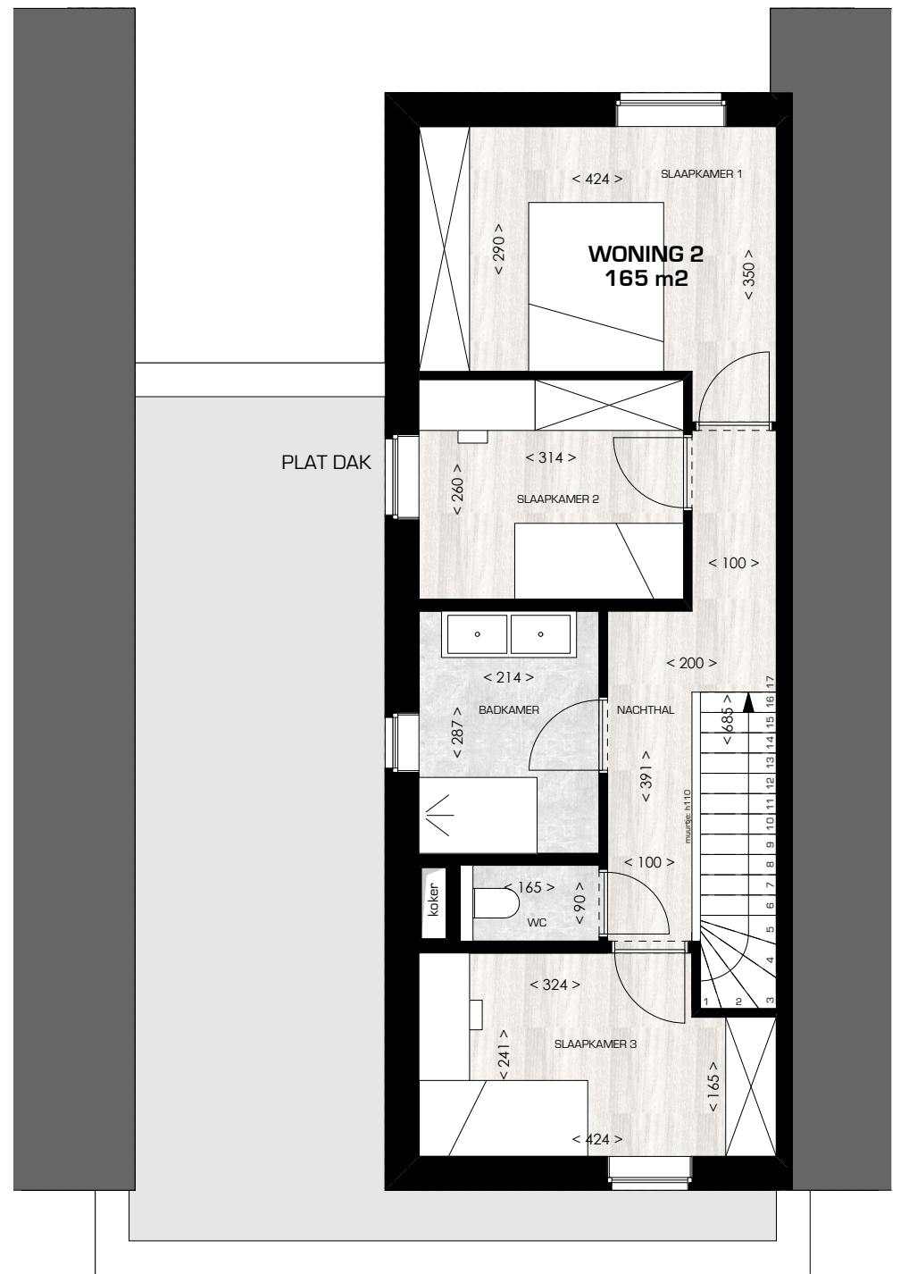
VERDIEPING
