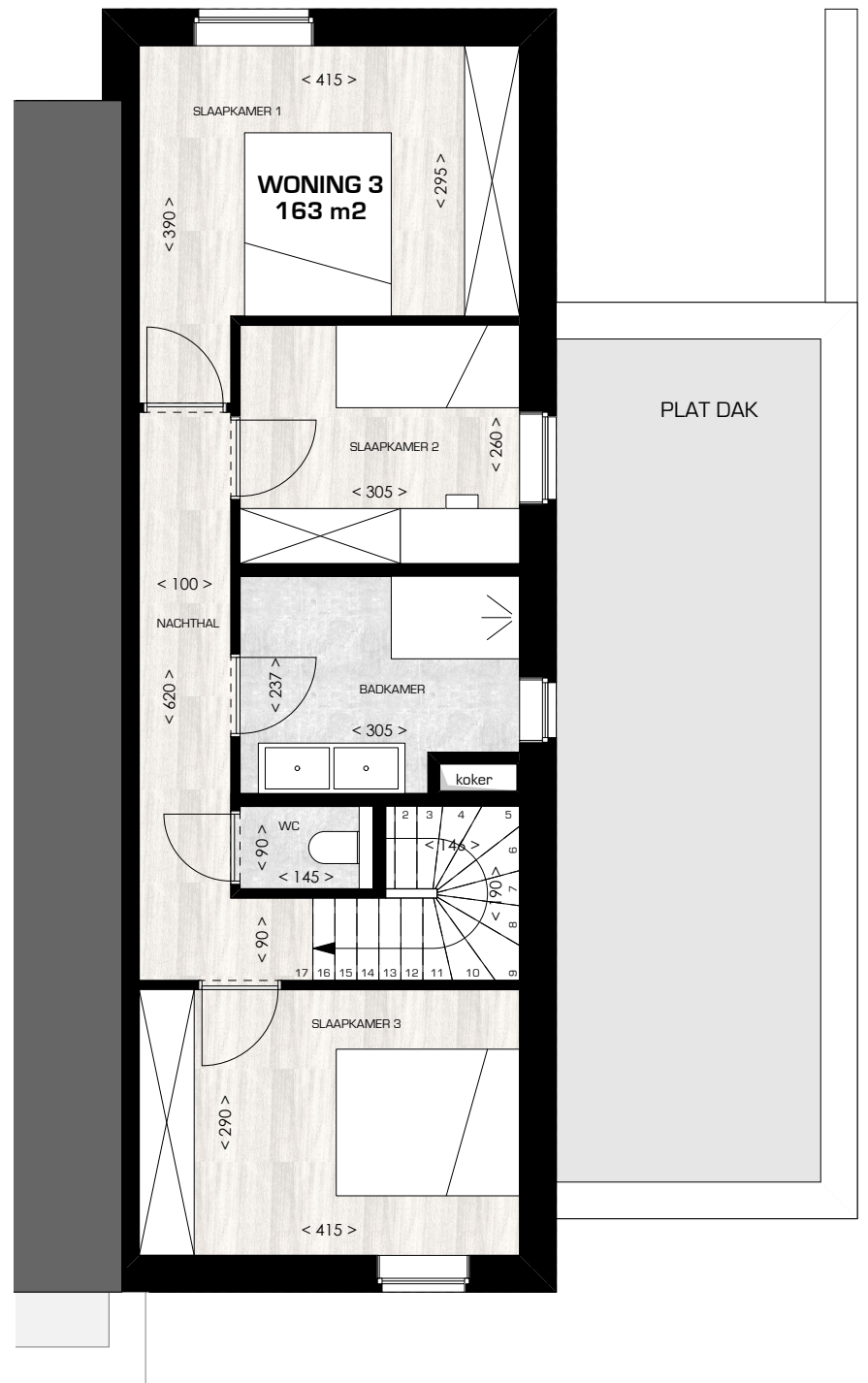
VERDIEPING
